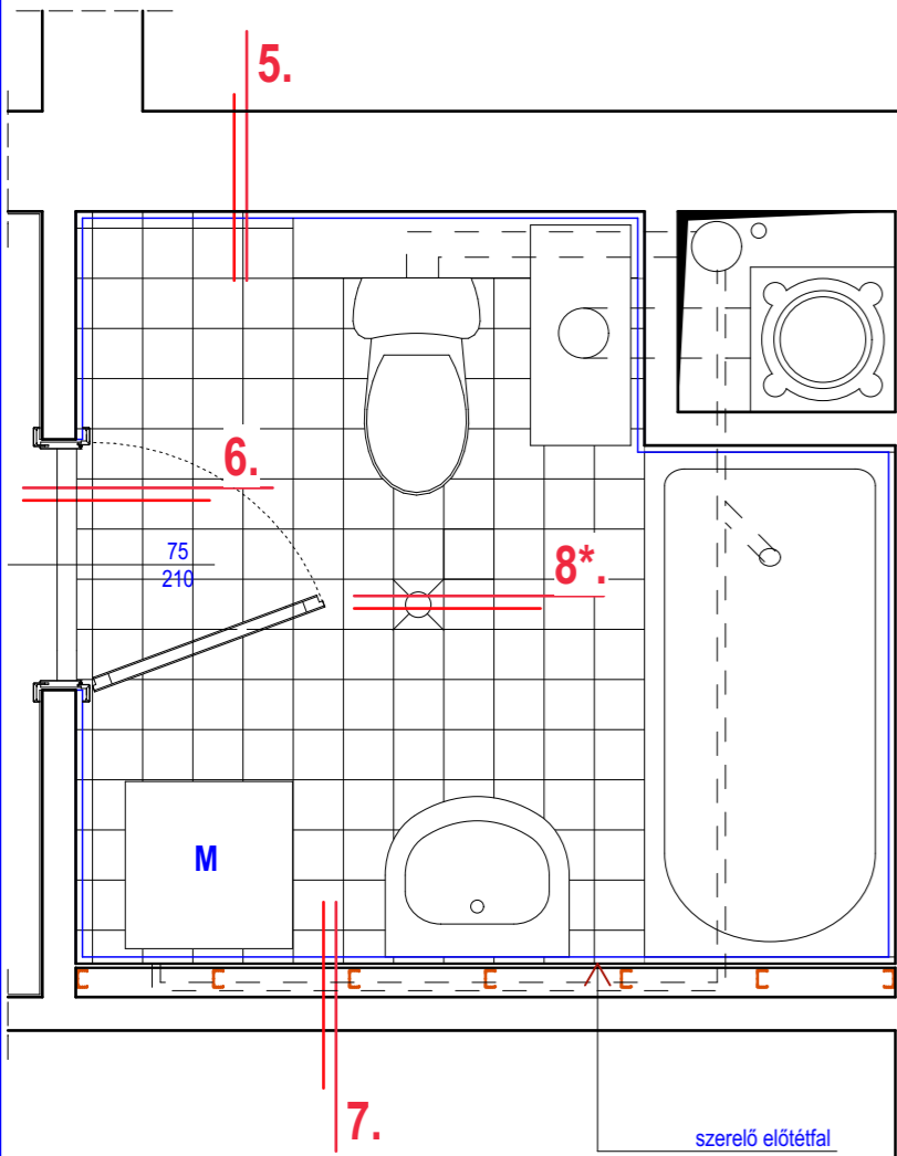
Alaprajz M=1:25
